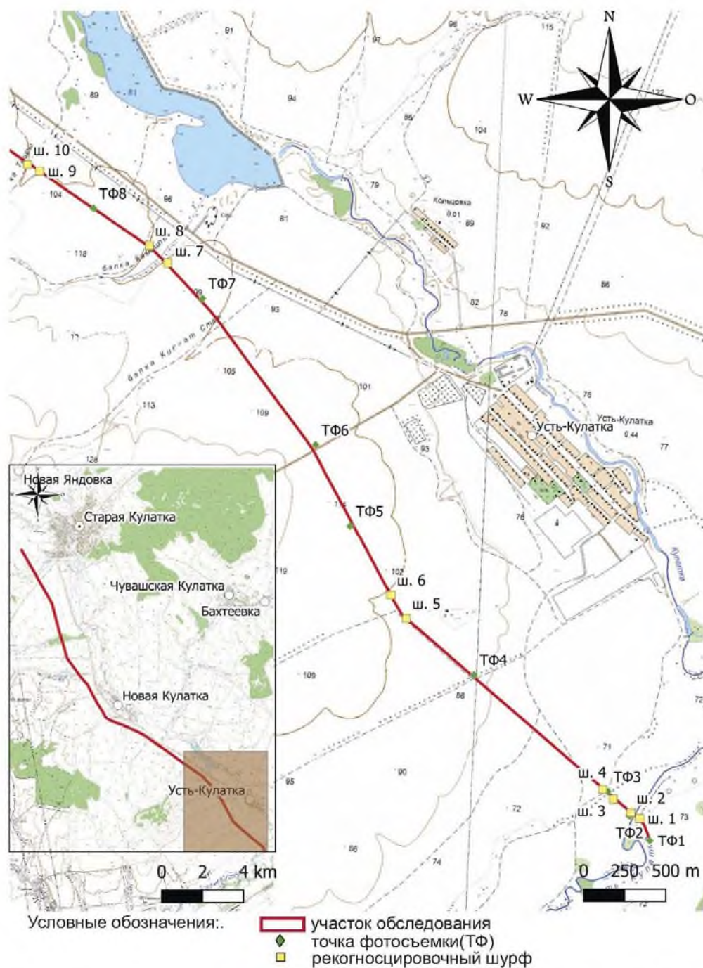
Илл.6. Схема расположения обследуемого объекта «Газопровод-отвод к ГРС-129 р.ц. Старая Кулатка (капитальный ремонт газопровода-отвода к г. Хвалынский, Ду 250, участок 22,2-41,6 км) инв. № 026484, Павловское ЛПУ км)» на территории Старокулаткинского района Ульяновской области.
